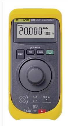
Obr. 1. Kalibrátor Fluke 707
