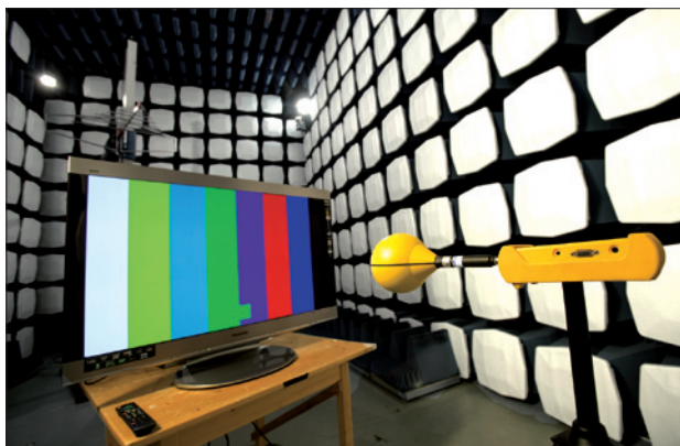
Obr. 1. Měření magnetického pole televizoru podle normy EN 50371 v laboratoři EZÚ, kterým se ověřuje ochrana člověka před účinky magnetického pole.
