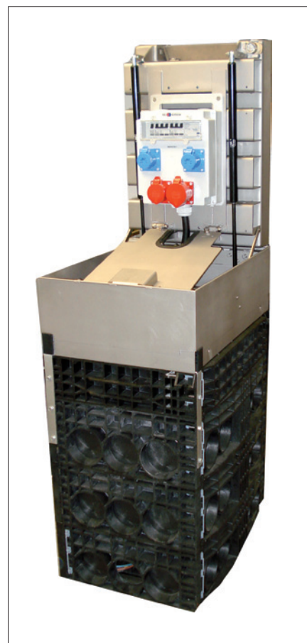
Obr. 3. Rozvaděč LIC před zapuštěním do země
