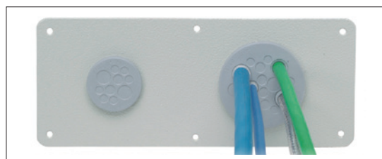
Obr. 1. Kulaté membránové průchodky KEL-DP
