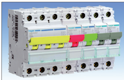
Obr. 1. Nová řada jističů s barevným rozlišením ovládacích páček dle jmenovitých proudů přístrojů u 1pólového a 3pólového provedení
