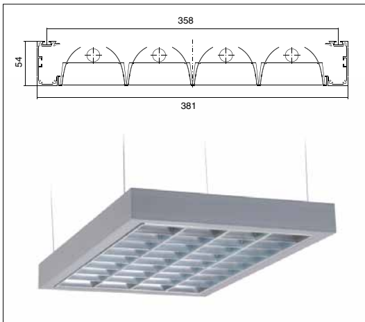
Obr. 1. Svítidlo Lambda
