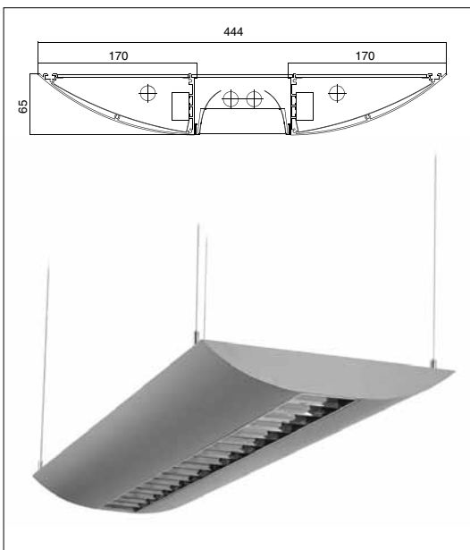
Obr. 2. Svítidlo Delta-T
