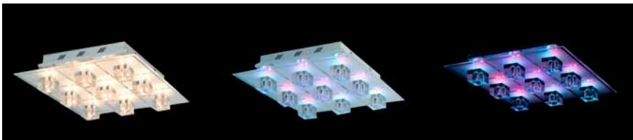
Obr. 2. WOFI – stropní svítidlo Zixi obj. číslo: WO 9933.09.06.0000, provedení: sklo křišťál a mat světelný zdroj: 9x halogenová žárovka 20 W, 12 V, G4, + 9x LED RGB (měnič barvu) dodáváno včetně světelných zdrojů, rozměry: 62 x 62 cm, výška 12 cm, cena včetně DPH: 16 164 Kč
