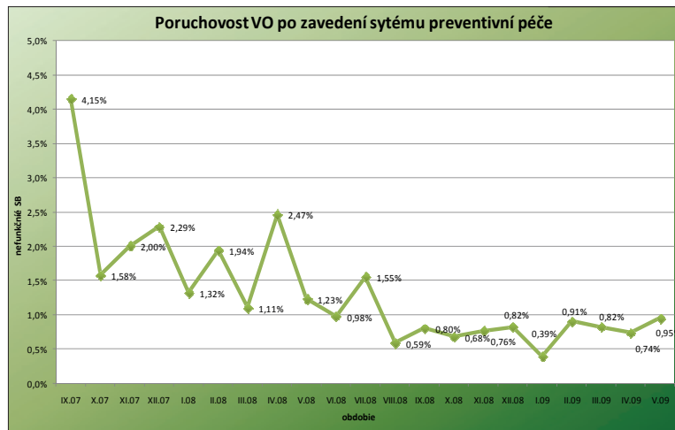
Obr. 1. Zníženie poruchovosti zariadenia verejného osvetlenia v meste Košice vďaka zavedeniu systému preventívnej starostlivosti a operatívnej údržby
