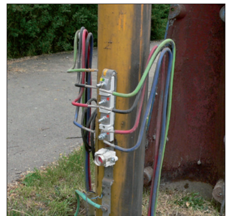
Obr. 4. Elektrovýzbroj verejného osvetlenia po prevedení preventívnej starostlivosti
