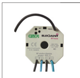
Obr. 3. Stmívací jednotka - přijímač
