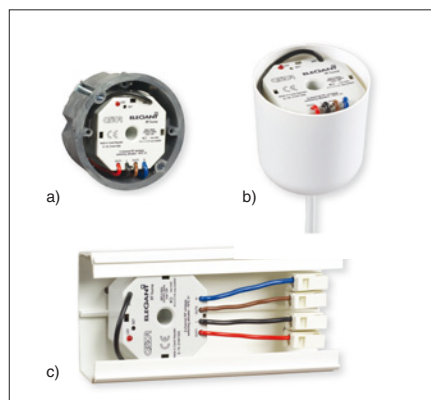
Obr. 4. Příklady montáže a) montáž přijímače do instalační krabice, b) montáž přijímače do stropního krytu svítidla, c) montáž přijímače do kabelových žlabů a kanálů
