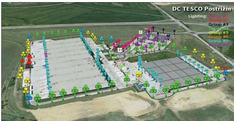
Obr. 2. Virtuální letecký pohled na venkovní osvětlení distribučního centra Tesco Postřizín; rozdělení osvětlení do skupin
