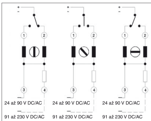
Obr. 2. Schémata připojení
