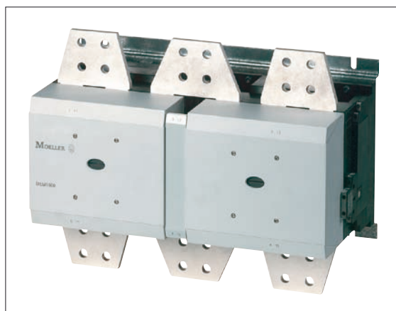
Obr. 3. Výkonový stykač DILM2000 pro spínání ohmických zátěží
