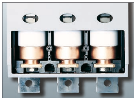
Obr. 1. Vakuové spínací komory
