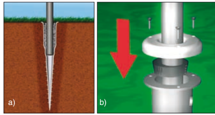
Obr. 8. Kolmost trubkového sloupku je v zemním vrutu upravena až po jeho zasazení do země a) vycentrováním obzvláště tvrdým a drsným ostrohranným lámavým granitovým štěrkem, b) patentovaným centrovacím systémem pro přesné nastavení
