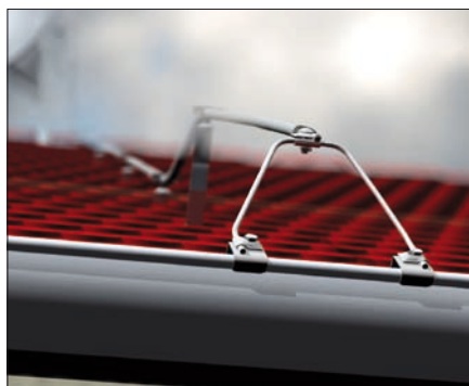
Obr. 5. Uchytení konce vodiče na okap
