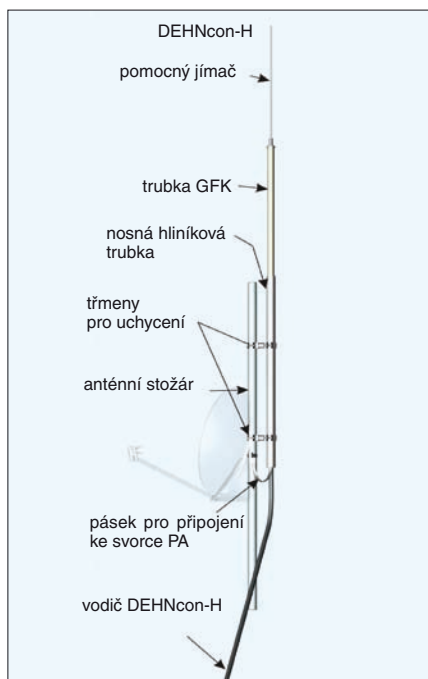
Obr. 2. Vodič HVI-light uložený v nosné trubce
