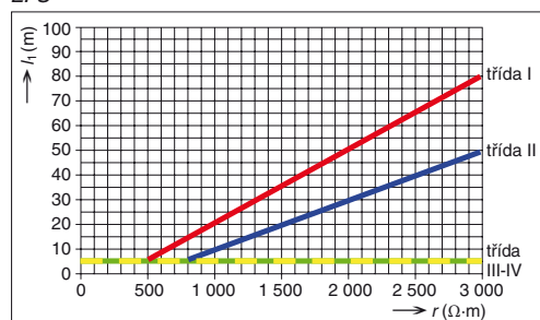
Graf minimální délky l_1 každého zemniče podle třídy LPS
