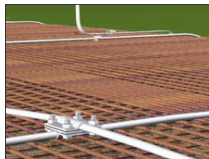
Obr. 8. Dráty a pásky uložené přes armovací rošt
