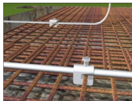
Obr. 9. Svorky pro jednoduché připojení armovacích prutů
