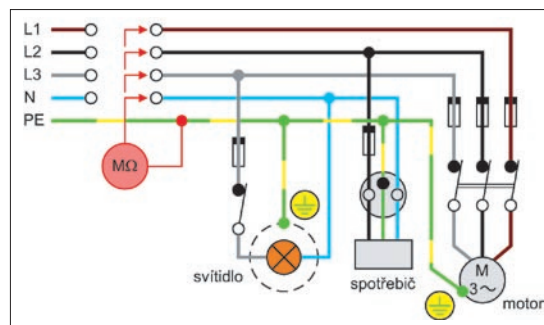
Příklad elektrického schématu měření izolačních odporů všech vodičů proti ochrannému vodiči PE
