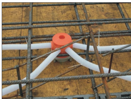
Obr. 6. Příklad použití na horizontálním bedněni
