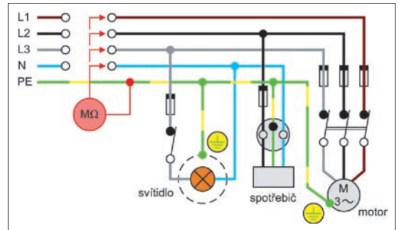
Příklad elektrického schématu měření izolačních odporů všech vodičů proti ochrannému vodiči PE
