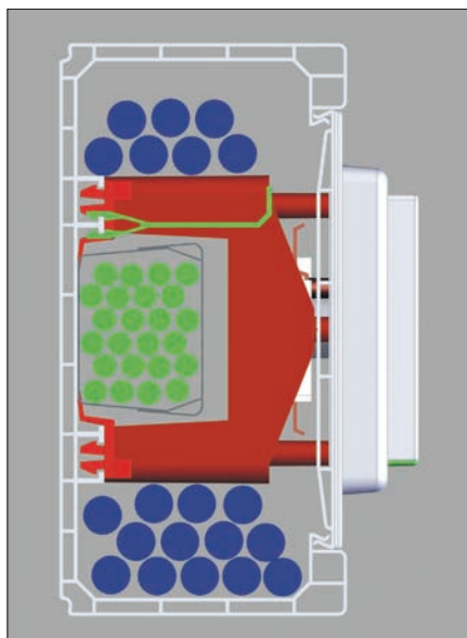
Obr. 5. Příklad uložení kabelů v kanálu PK 140 × 70 D
